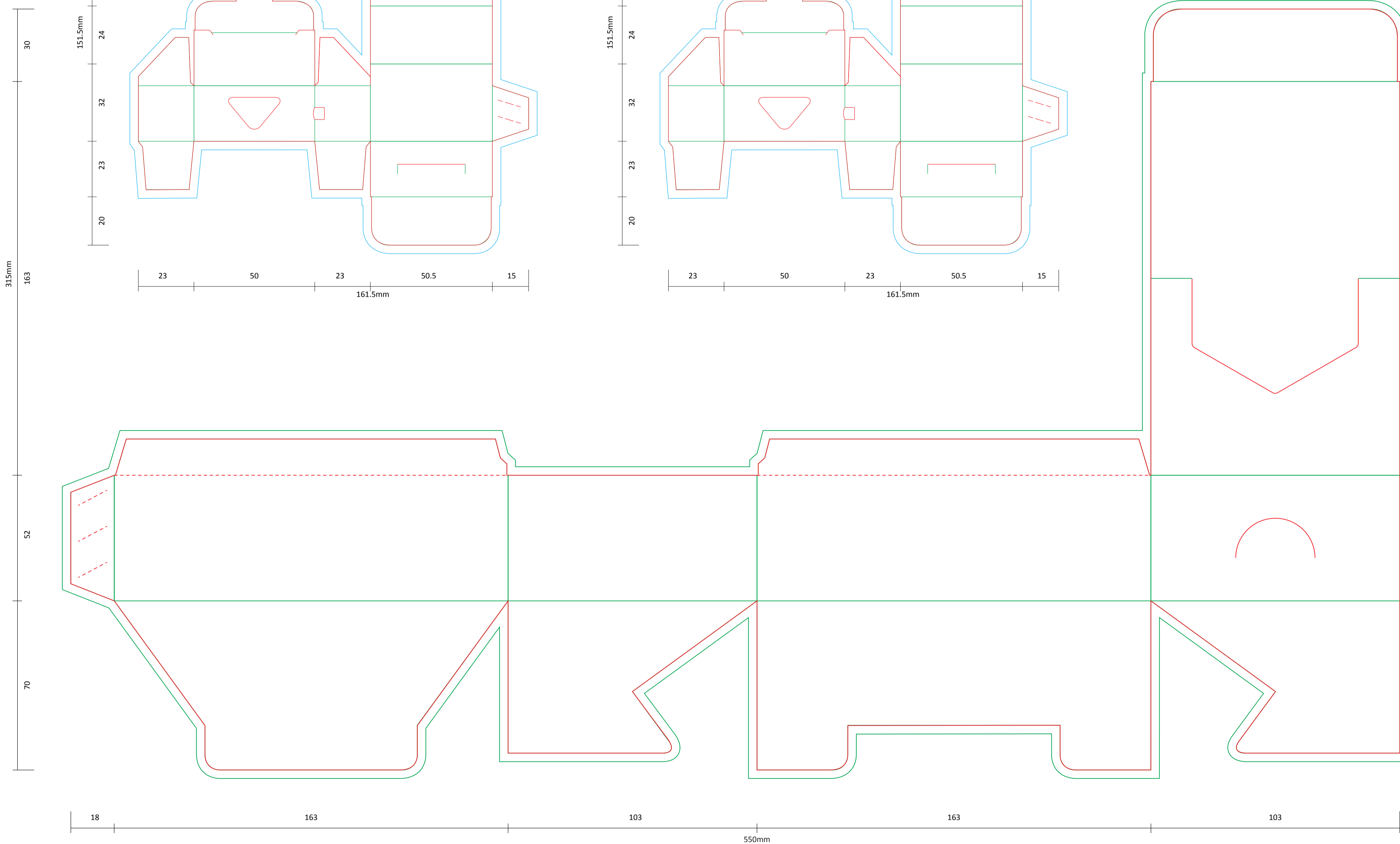
DISPLAY BOX - 20 PACKS/BOX
